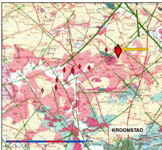
Abbildung 19: Karte nördlich von Kroonstad. Punkte markieren Kimberlit-Cluster. Pfeil zeigt auf Voorspoed Mine (Vortrag Powerpoint).
