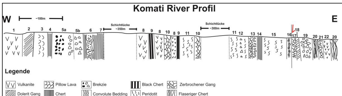
Abb. 4: Komati River Profil (umgezeichnet, nach Feldbuchskizze Lammerer, nicht maßstäblich)
